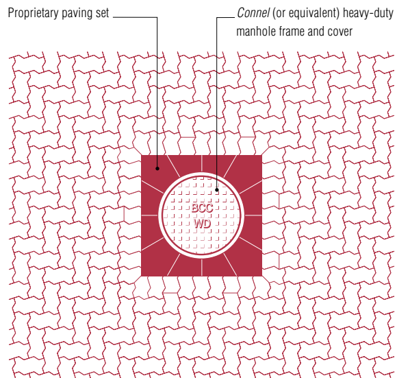
Manhole paving set
